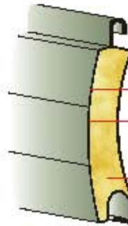
Poliüretan dolgulu pvc kaplı çelik palet
