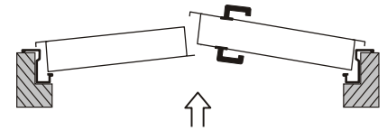
Çift kanatlı kapı - Sağ Yön Açılım (DX)
