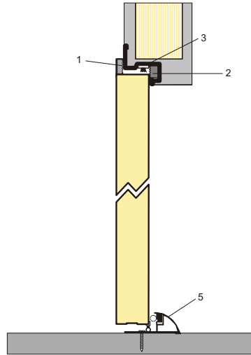
DETAY PP2 (Kit KA4)
