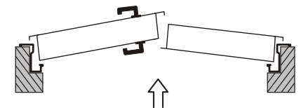
Çift kanatlı kapı - Sol Yön Açılım (DX)
